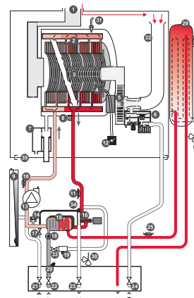
Schema funzionale
